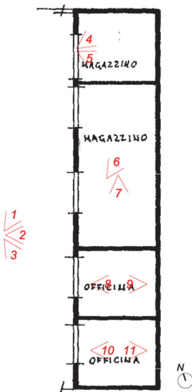
Planimetria fabbricato servizi con indicazione dei punti di presa delle foto seguenti
